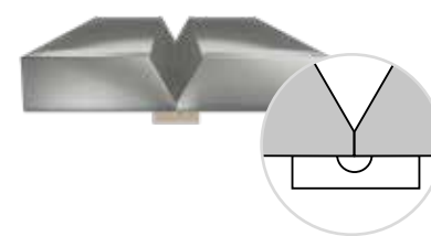
Nahtvorbereitung ohne Luftspalt
