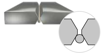
Zylindrische / runde keramische Badsicherung, Durchmesser abhängig von Nahtvorbereitung und Luftspalt
