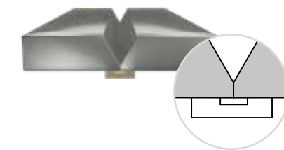
Nahtvorbereitung ohne Luftspalt
