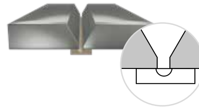
Nahtvorbereitung mit Luftspalt
