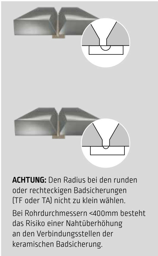
Nahtvorbereitung ohne Luftspalt
