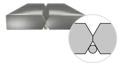
X-Nahtvorereitung ohne Luftspalt
