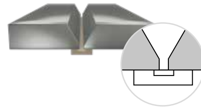
Nahtvorbereitung mit Luftspalt
